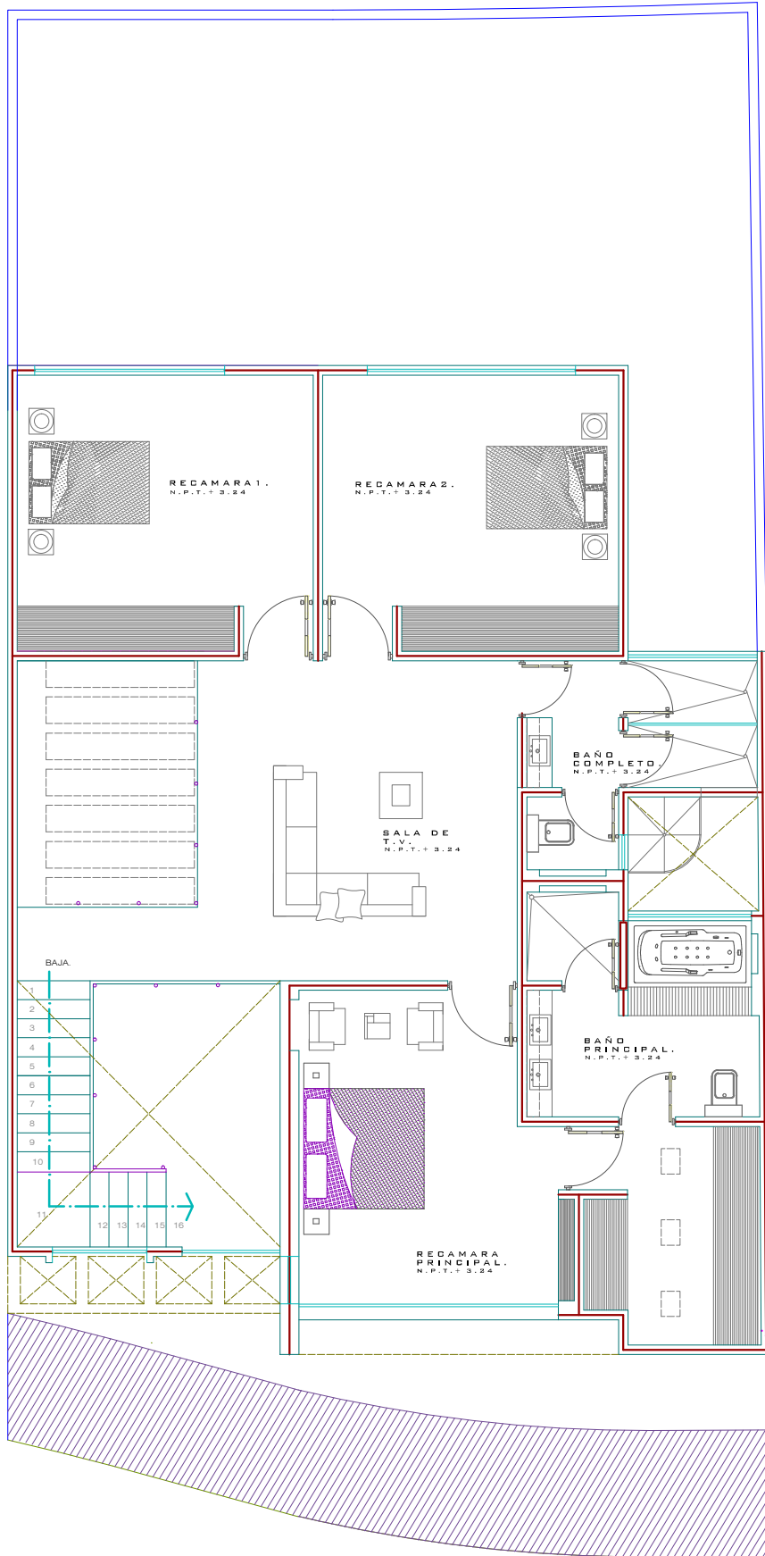
PLANTA ARQUITECTONICA ALTA
