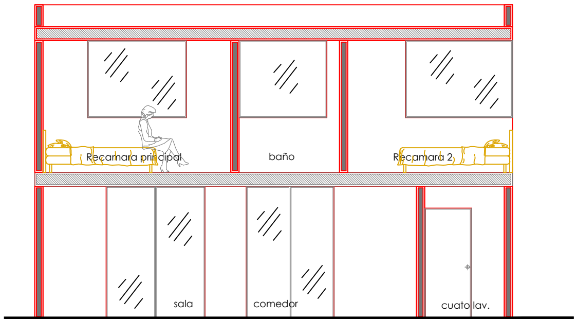
CORTE bb'
