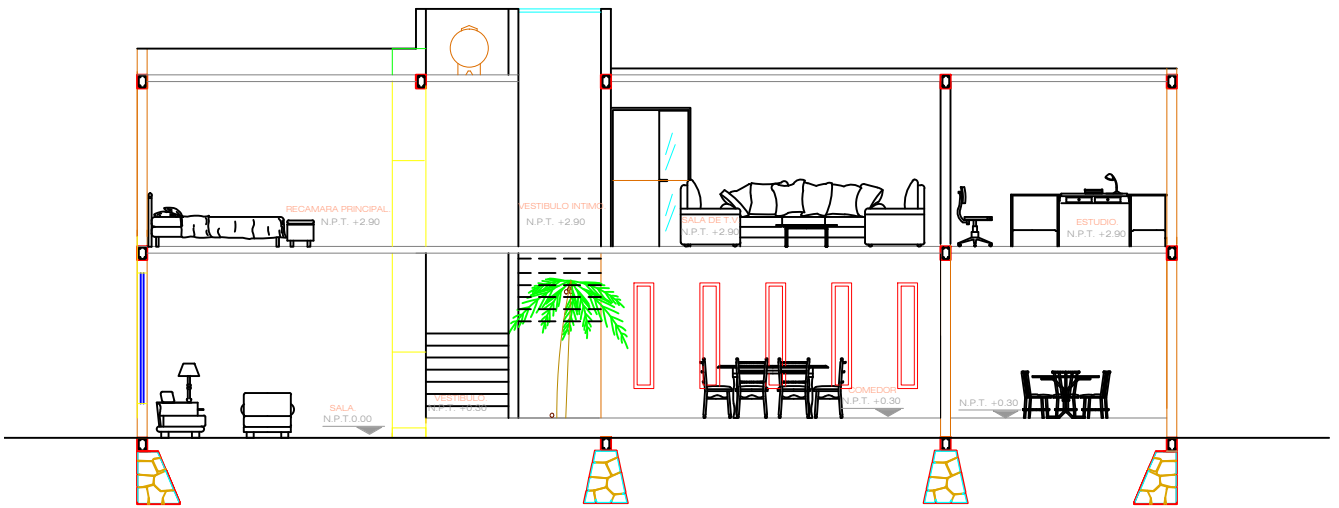
CORTE B-B'
