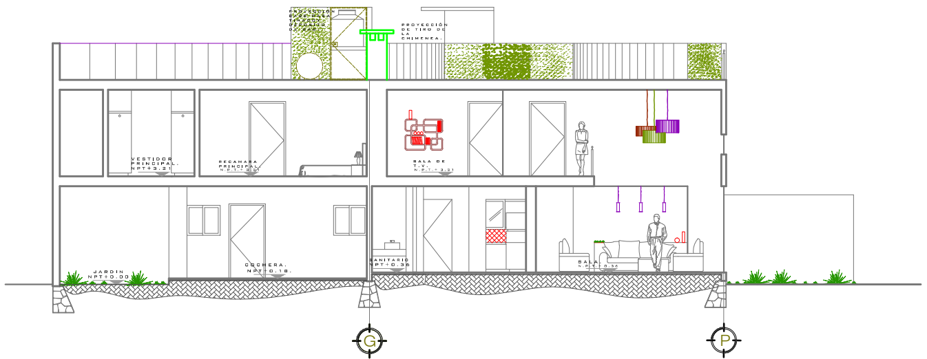
CORTE X-X'.
